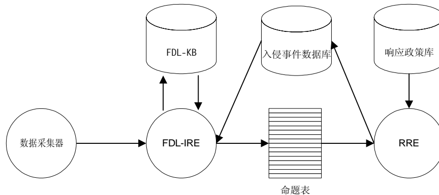
图2 FDL-IDS系统框架
