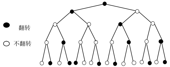
图3 匿名化函数树
