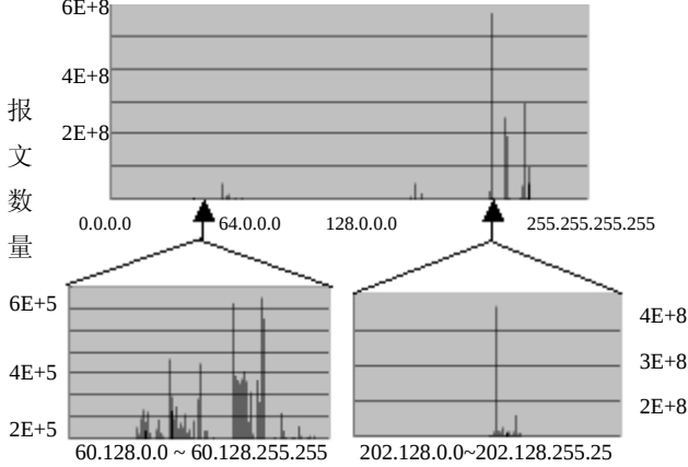
图2 原始数据集中 IP 地址对应的报文数量分布 Fig.2 The distributing of IP addresses and packet number
